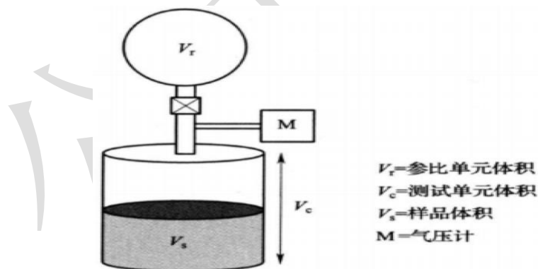
图 气体置换法真密度仪原理图
